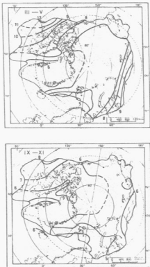
Ryc. 3b. Średnie sezonowe (III-V i IX-XI) dobowe amplitudy temperatury powietrza (w °C) w Arktyce w okresie 1951-1990.
