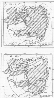
Rys. 5. Trendy średnich sezonowych (XII-II, III-V, VI-VIII i IX-XI) dobowych amplitud temperatury powietrza (w °C/10 lat) w Arktyce w okresie 1951-1990
