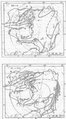
Ryc. 3a. Średnie sezonowe (XII-II i VI-VIII) dobowe amplitudy temperatury powietrza (w °C) w Arktyce w okresie 1951-1990.
