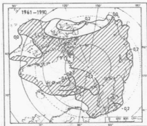
Ryc. 4. Trendy średnich rocznych dobowych amplitud temperatury powietrza (w ^{\circ}\text{C}/10 lat) w Arktyce w okresach: 1951-1990, 1961-1990 i 1971-1990.
